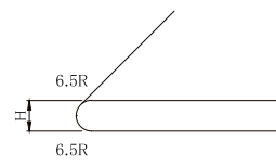
ボウズ面取
